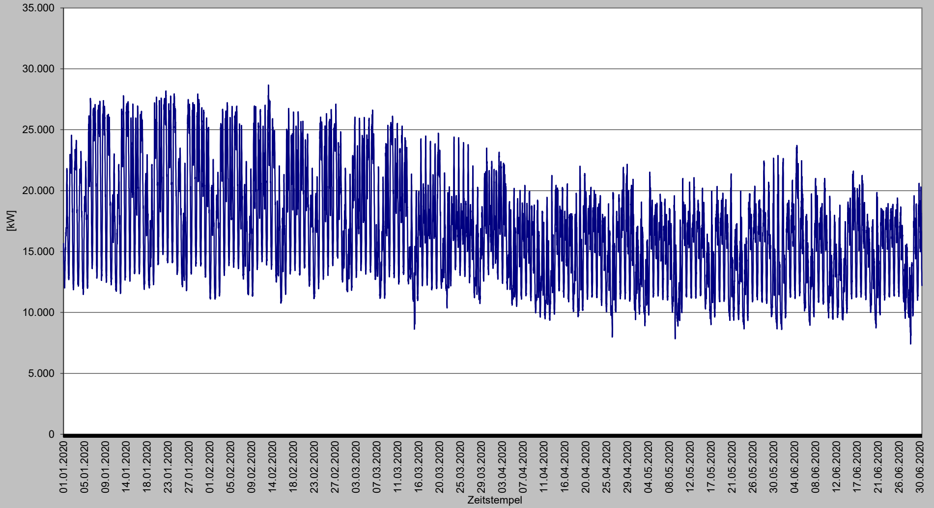
Lastverlauf im Verteilnetzgebiet der Stadtwerke Dülmen GmbH im 1. Halbjahr 2020
