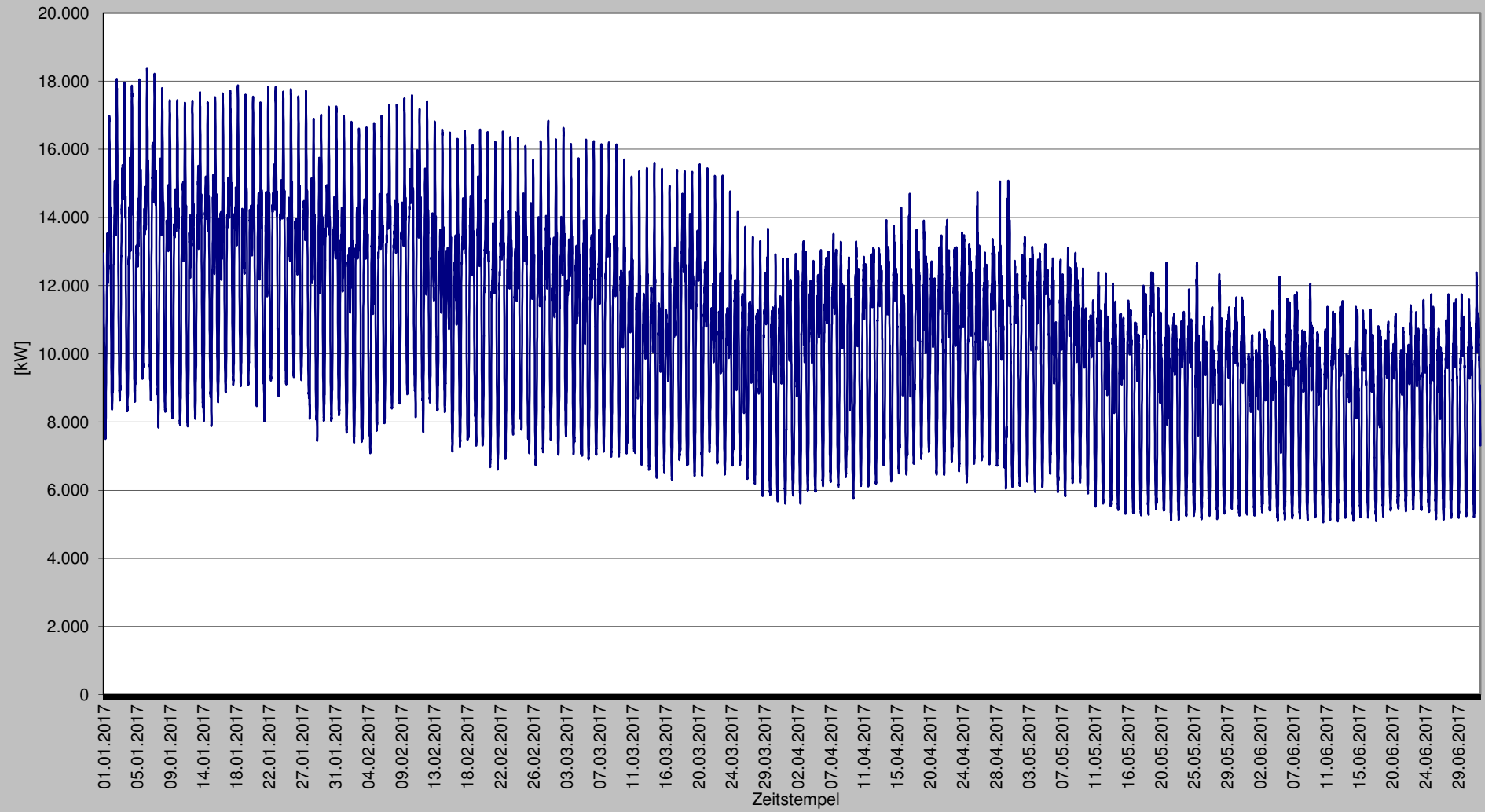
Lastverlauf Nsp. - oL. im Netzgebiet der Stadtwerke Dülmen GmbH für das 1. Halbjahr 2017
