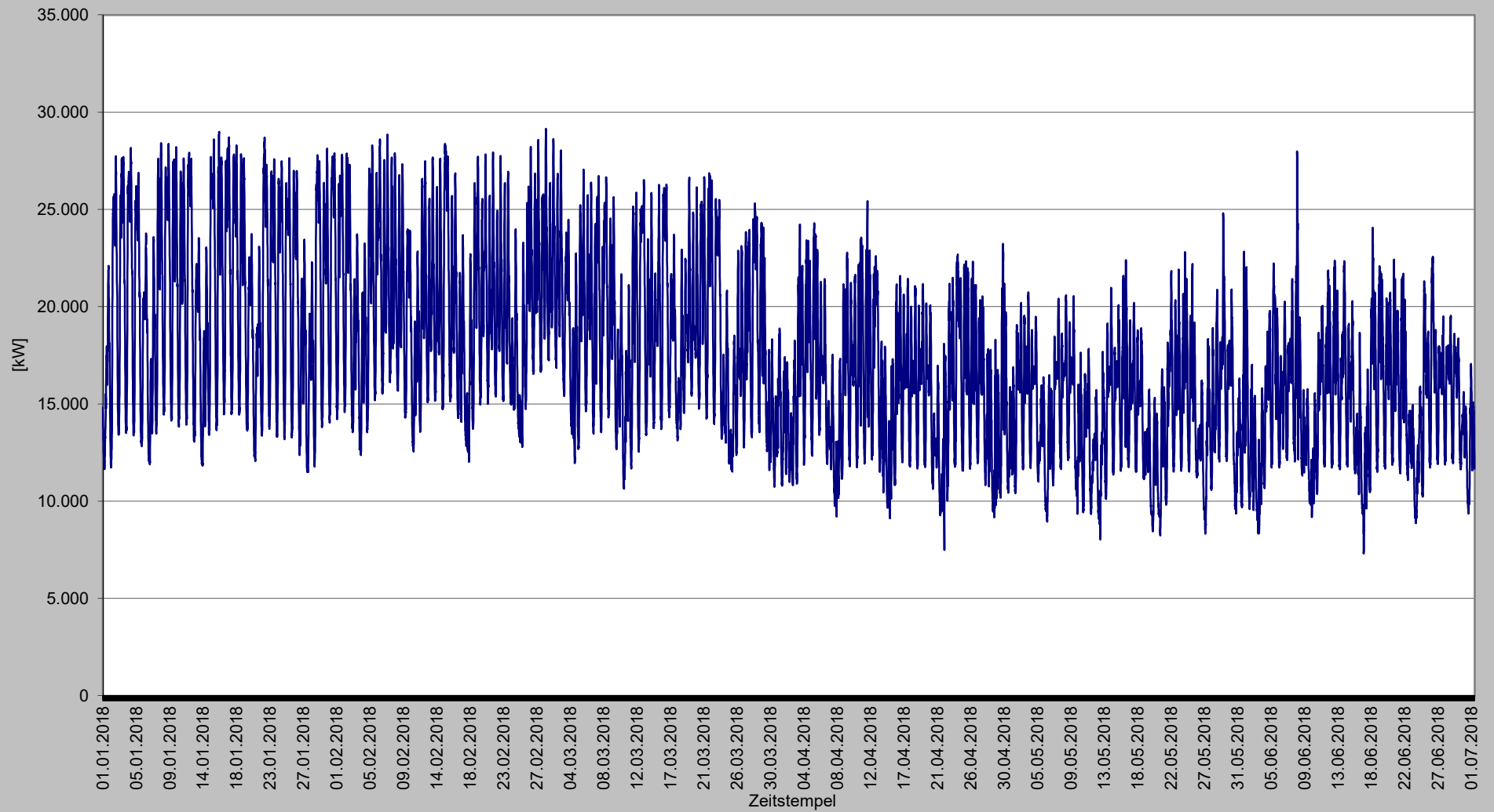
Lastverlauf im Verteilnetzgebiet der Stadtwerke Dülmen GmbH im 1. Halbjahr 2018
